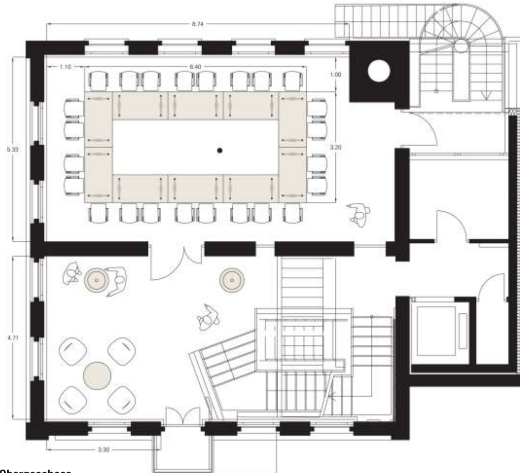
Mahlwerk - 1. Obergeschoss
